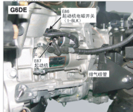
54. 发动机前部
