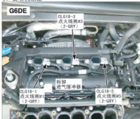
50. 发动机顶部
