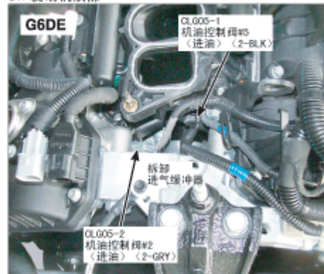
51. 发动机顶部
